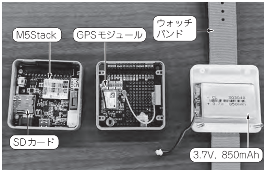
写真1 実験に使用したハードウェア…IoTマイコンESP32を内蔵するM5Stackは数センチ角の機能モジュールを複数お好みで積み重ねられる ここではM5Stackメイン基板とGPSモジュール、ウォッチバンドの3つを用意した
