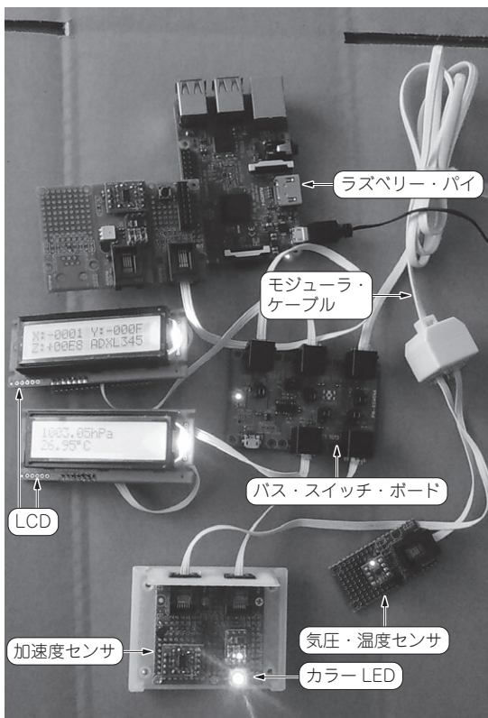
(a) ラズベリー・パイとさまざまなI/Oモジュール
