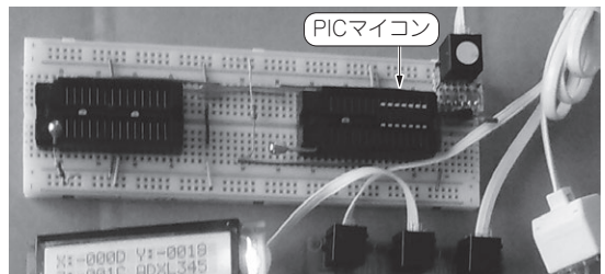
(b) PICマイコンの接続例
