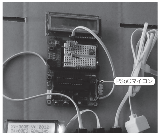
(c) PSoCマイコンの接続例
