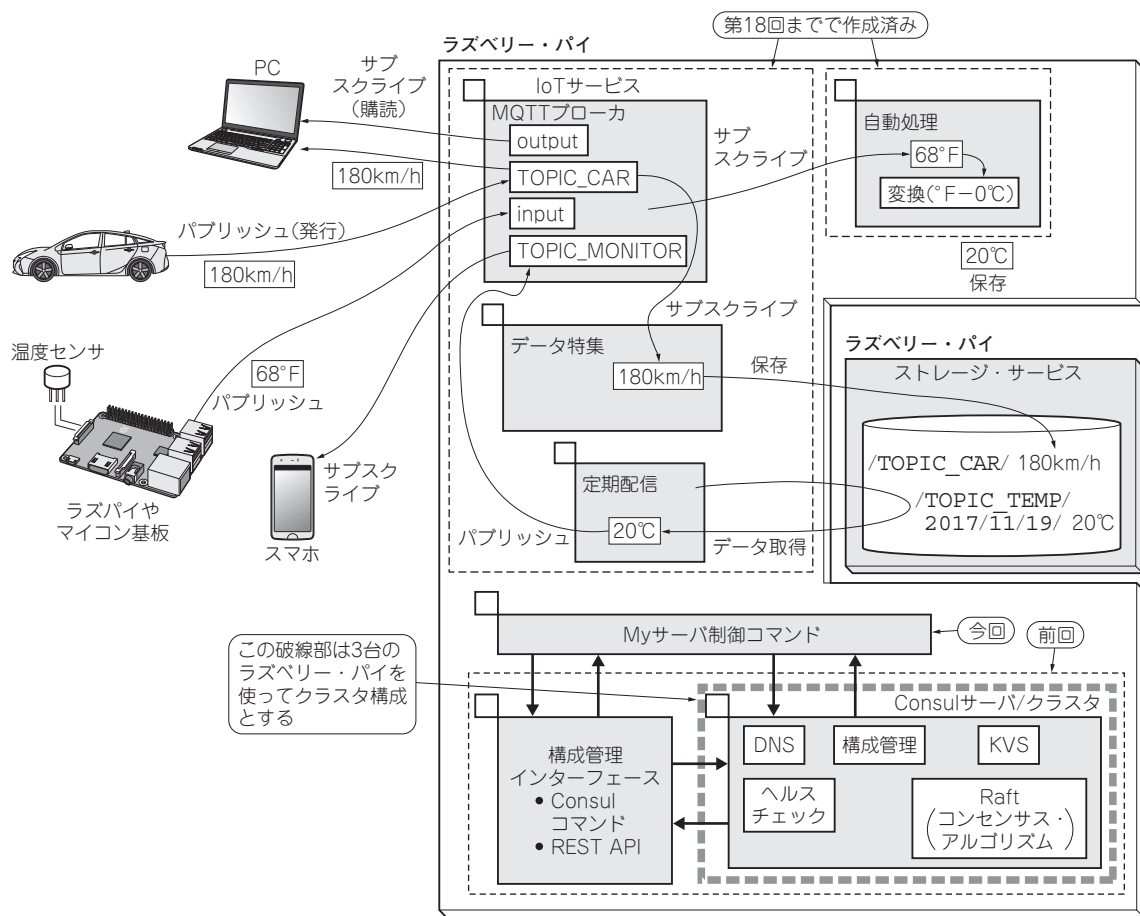
図1 ラズベリー・パイ上に構築したMyサーバのサービスを構成管理ソフトウェア Consulで管理する
