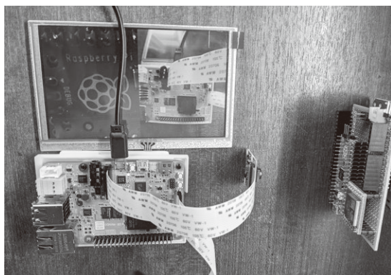
写真1 GR-MANGOはArm Cortex-A9「RZ/A2M」を搭載した、ラズベリー・パイ4の端子レイアウトと互換性があるボード
