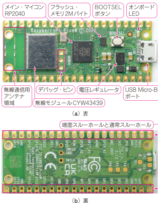
写真1 Pico Wの構成部品
