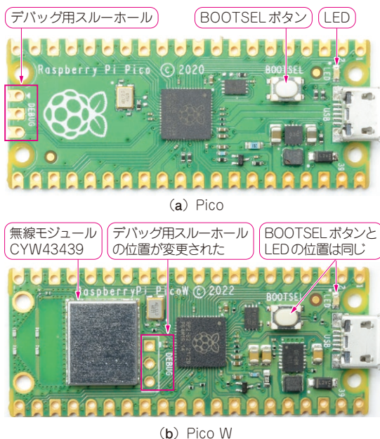
写真2 PicoとPico W搭載部品の位置関係
