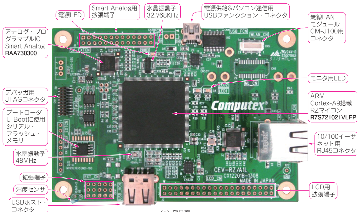
(a) 部品面
