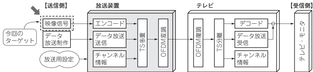
図2 デジタル放送の信号処理
