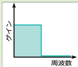
ローパス・フィルタ
