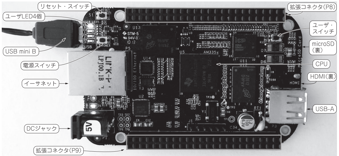
写真1 5000円で買える Cortex-A8 ボード BeagleBone Black
