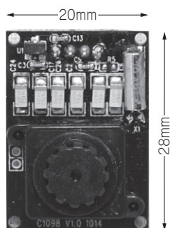
写真1 8ビット・マイコンからでもOKのJPEGシリアル出力カメラ C1098-SS
