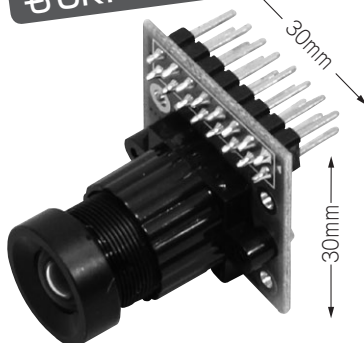
写真2 映画館の客席も映る! MT9V111カメラモジュール
