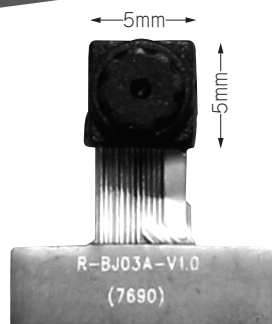
写真3 カメラ・ヘッド部分は5mm×5mm×3mmと小型! OV7690-FFC24P
