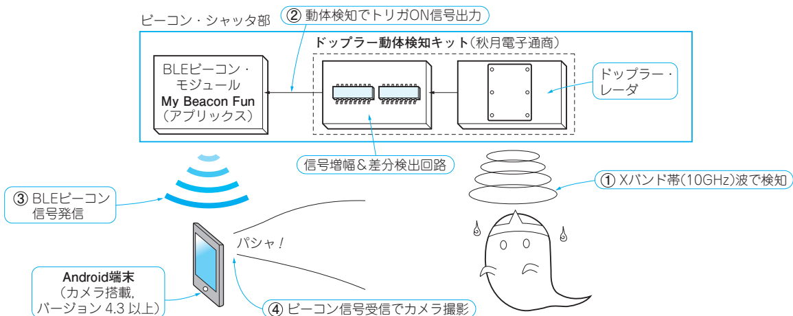
図1 複数のスマホから同時撮影もOK! BLE ビーコンを使った動体シャッター・カメラ・システム：幽霊が撮影できるかも…?
