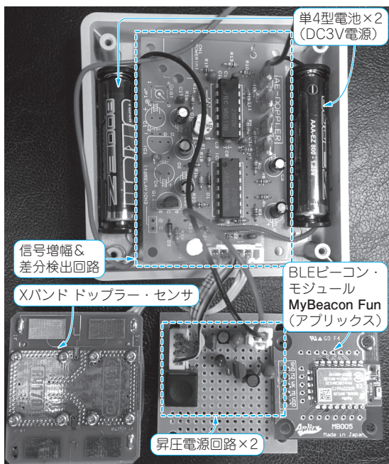
写真1 今回製作するBLEビーコン不審物カメラ(ビーコン・シャッター部)
