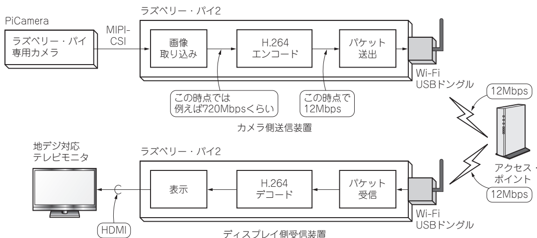
図1 データ送受信実験に用いた構成
