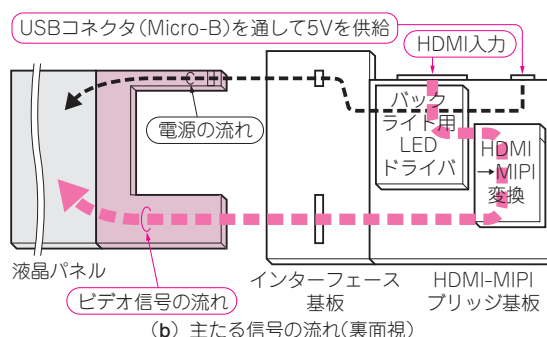
図1 キットには3枚の基板やパネルが入っている
