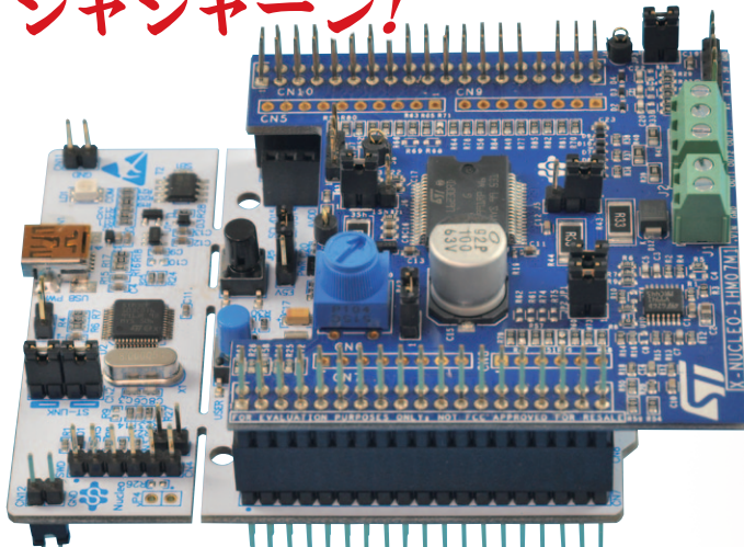
マイコン・メーカーが用意した価格破壊キット
